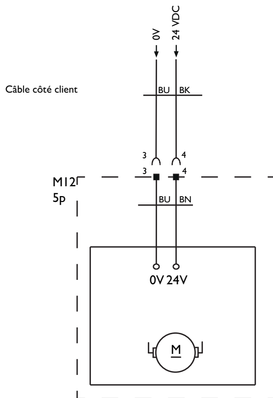
Fig. 3-1 Raccordement d'EPS
