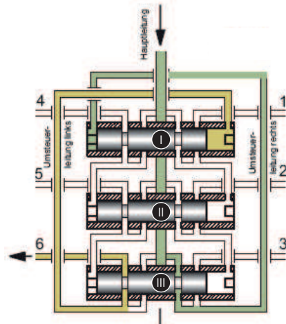
图 2-3 步进式分配器功能，图 1
