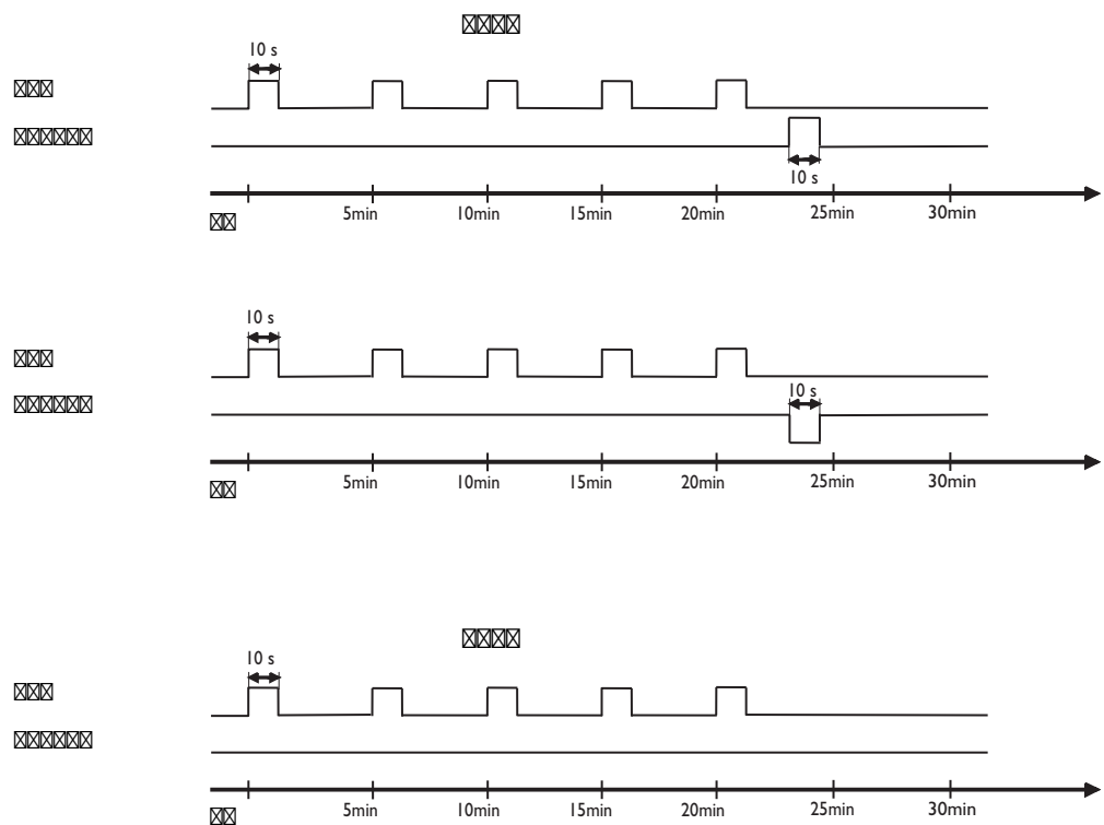
图 3-2 时序信号波形
