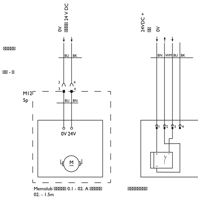
图 3-1 连接 PLCD
