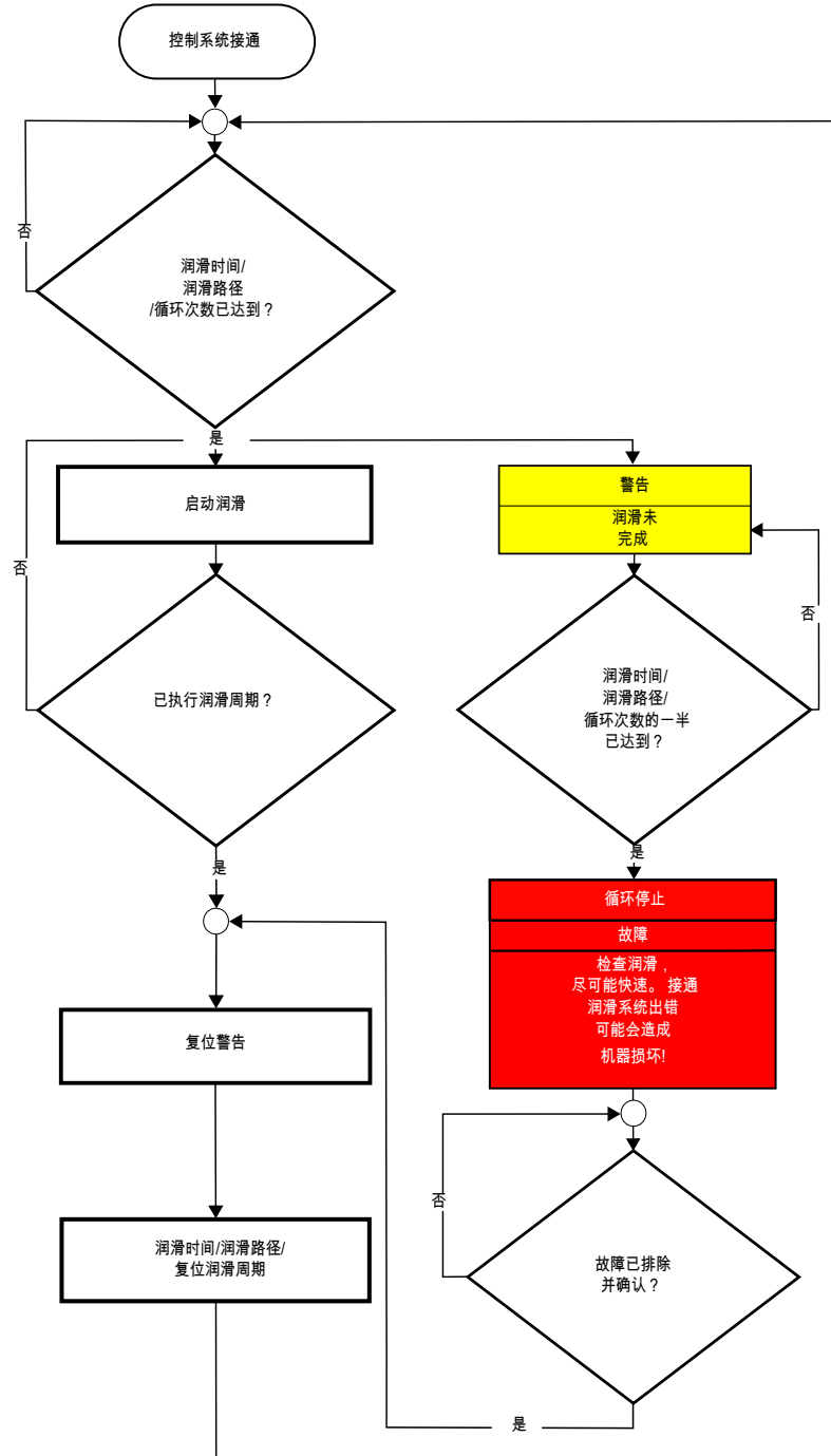
图 3-3 自动润滑装置流程图
