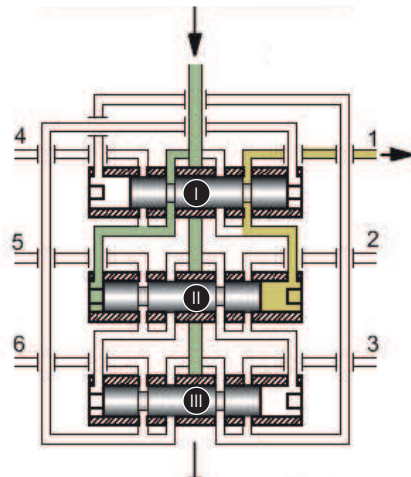
图 2-4 步进式分配器功能，图 2
