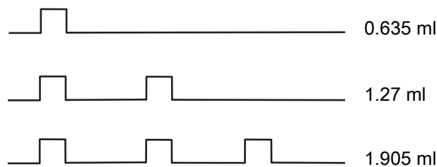
图 4-1 注油器处润滑量的计算示例
